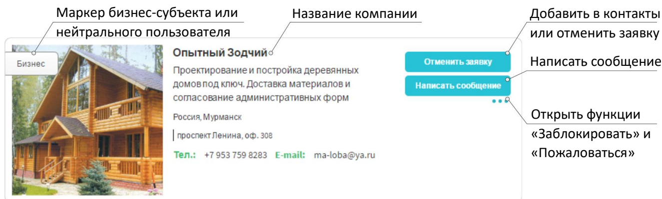
Рис. 1 – Карточка бизнес-субъекта
